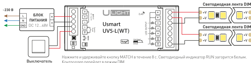
Рис. 1. Схемы подключения диммера USMART
