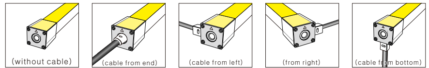
Cable outlet
