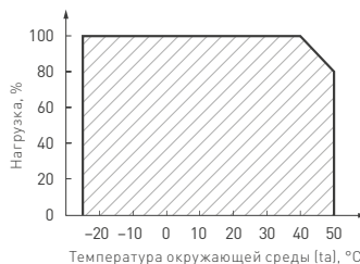
Рисунок 6. Максимальная допустимая нагрузка, % от мощности источника
