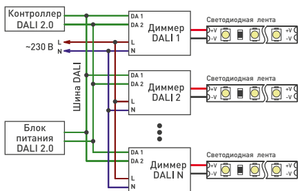
Рисунок 3. Схема подключения нескольких источников питания при использовании управления DALI 2.0
