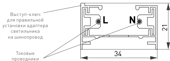
Рисунок 1. Конструкция шинопровода.
