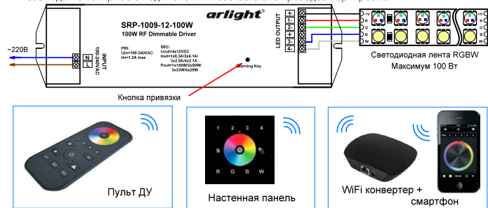
Рис.1. Подключение контроллера при использовании RGBW светодиодной ленты.
