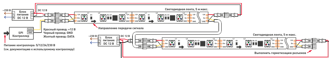
Рис. 2. Схема подключения лент SPI-5000P и SPI 2-5000PS.
