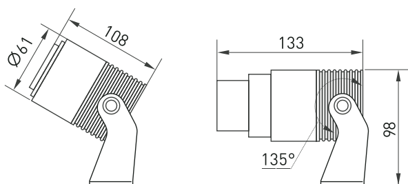
Рис. 1. Чертеж и габаритные размеры
